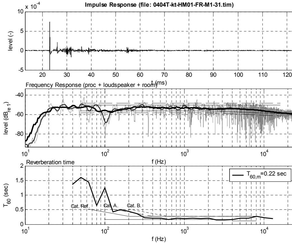
10. ábra: Mérési eredmények az FR-M1 átvitelből.
