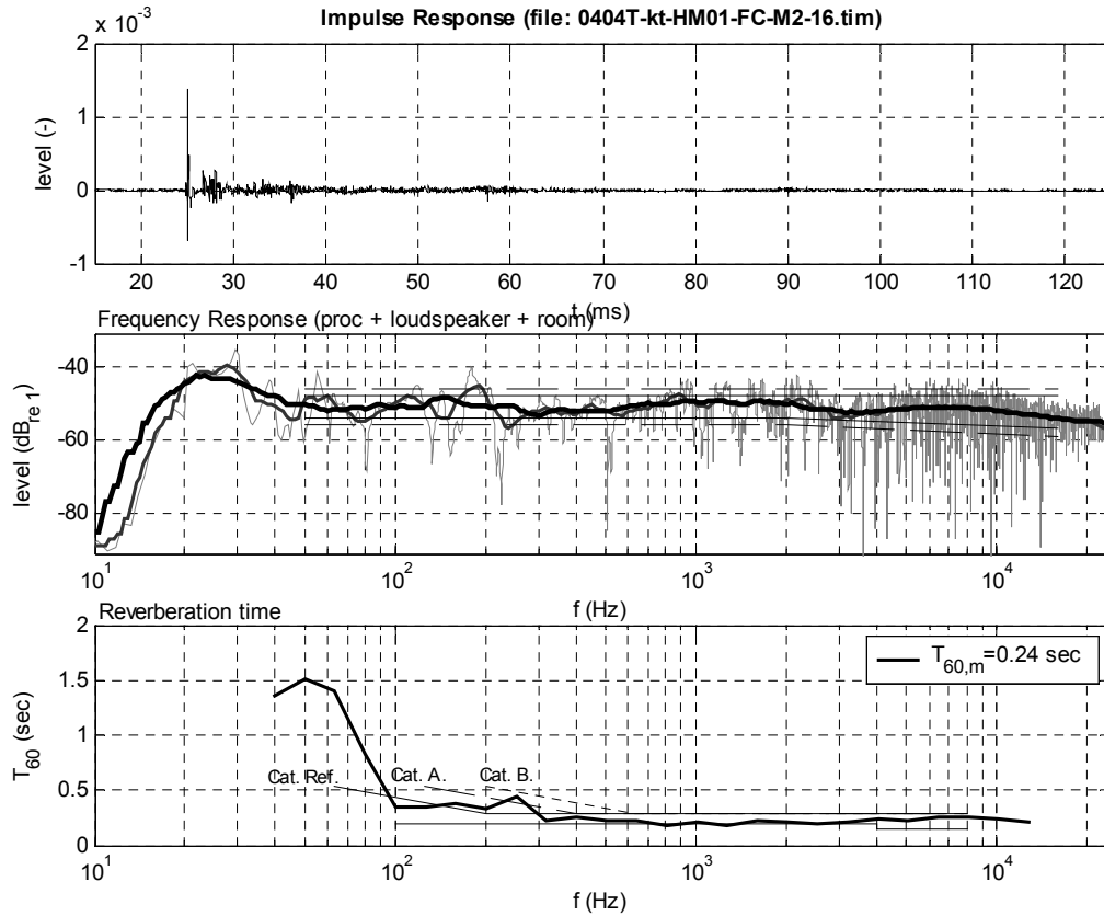
8. ábra: Mérési eredmények az FC-M2 átvitelből.
