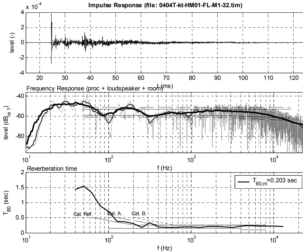
4. ábra: Mérési eredmények az FL-M1 átvitelből.
