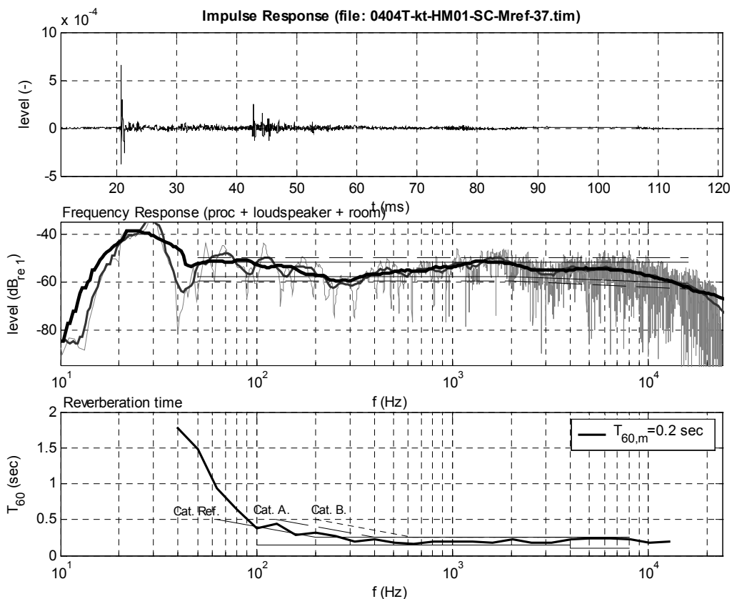
14. ábra: Mérési eredmények az SC-Mref átvitelhől.
