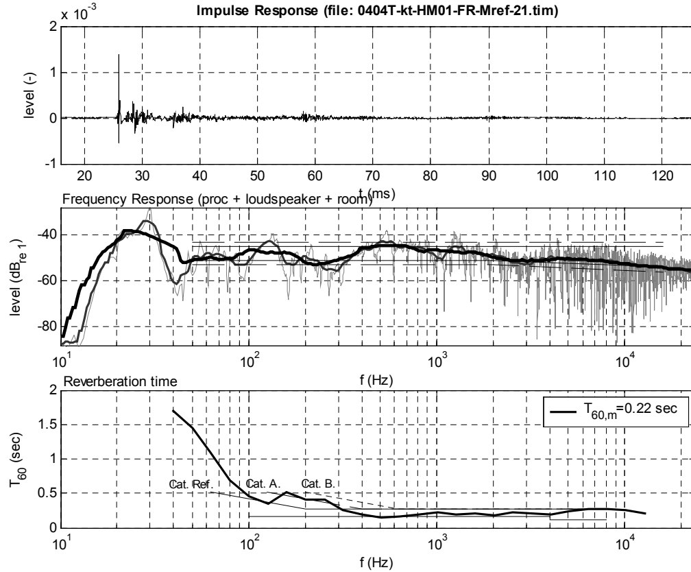
9. ábra: Mérési eredmények az FR-Mref átvitelből.
