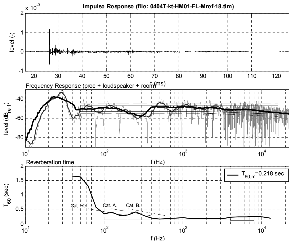
3. ábra: Mérési eredmények az FL-M ref átvitelből.
