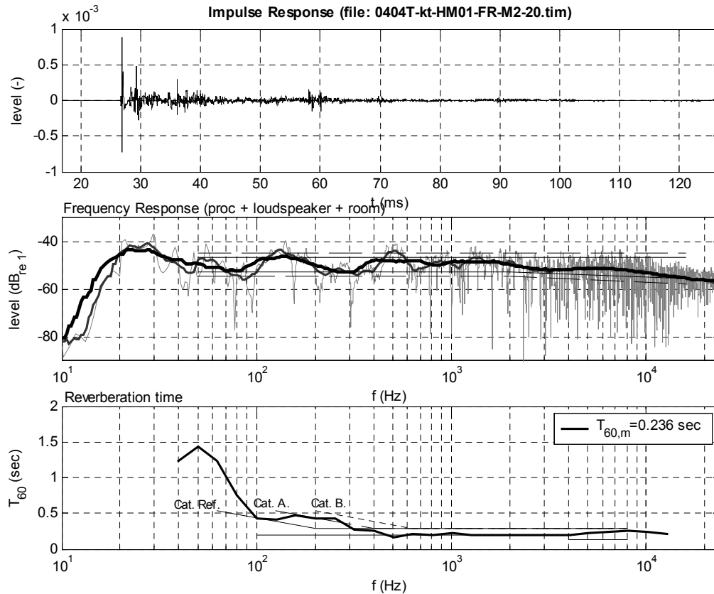
11. ábra: Mérési eredmények az FR-M2 átvitelből.
