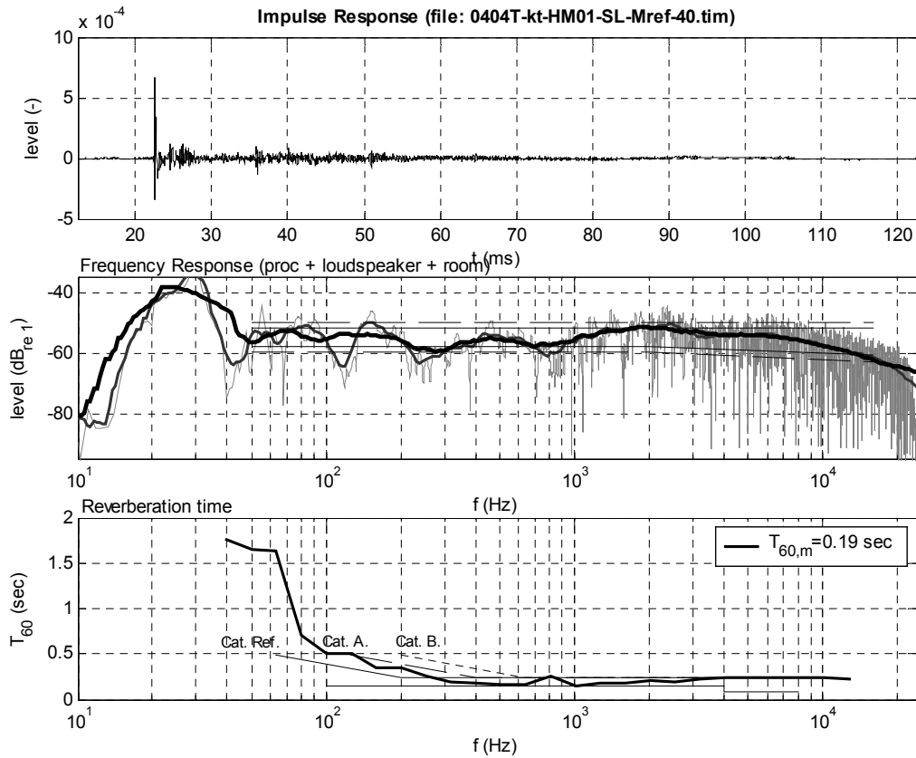
12. ábra: Mérési eredmények az SL-Mref átvitelből.
