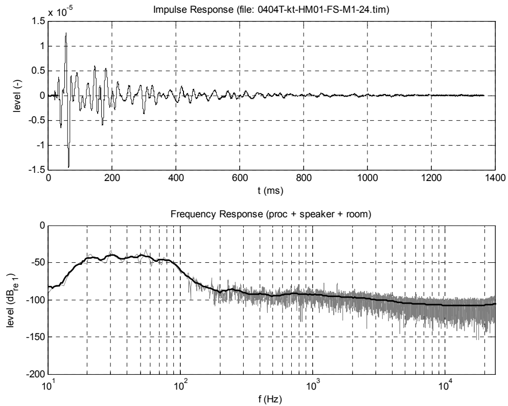
21. ábra: Mérési eredmények az FS-M1 átvitelből.
