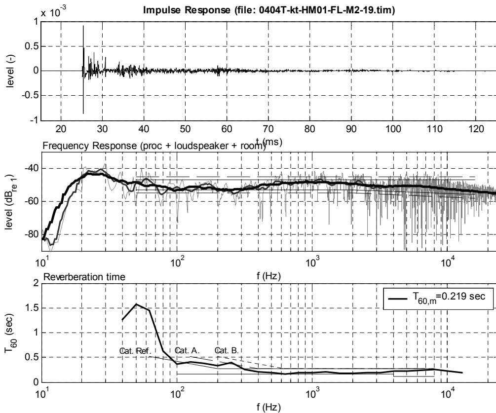
5. ábra: Mérési eredmények az FL-M2 átvitelből.
