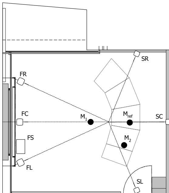
1. ábra: A mérési elrendezés; hangsugárzó és hallgatási pozíciók, elnevezéseik.
