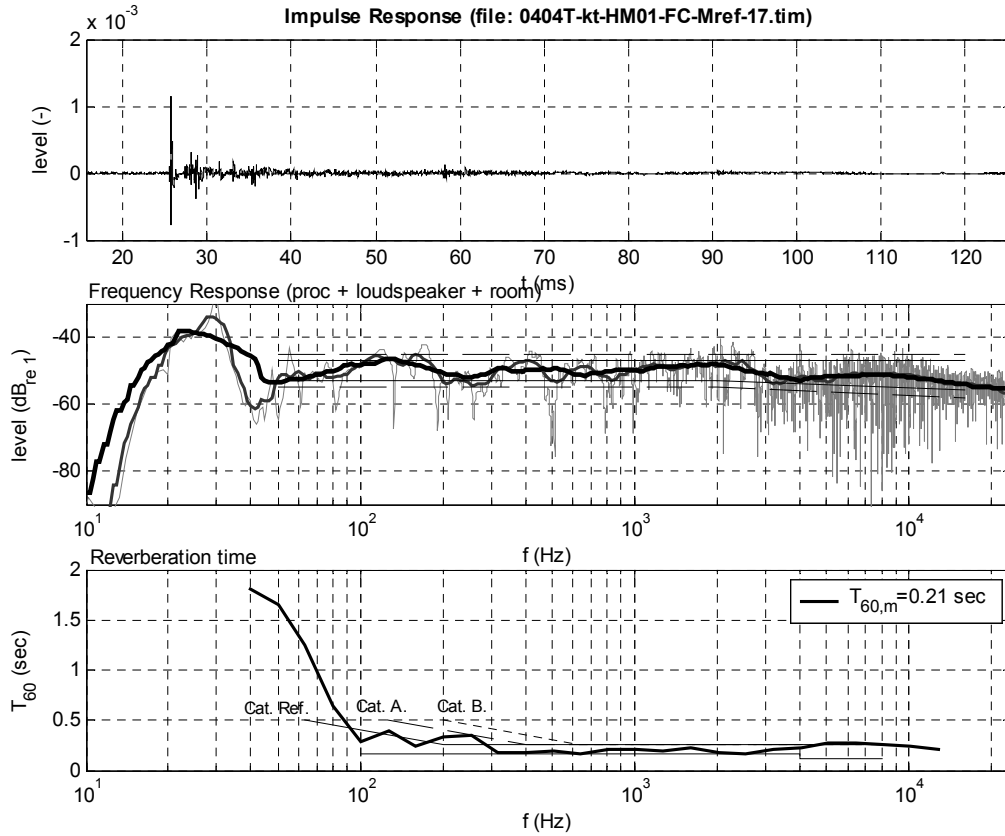
6. ábra: Mérési eredmények az FC-Mref átvitelhől.
