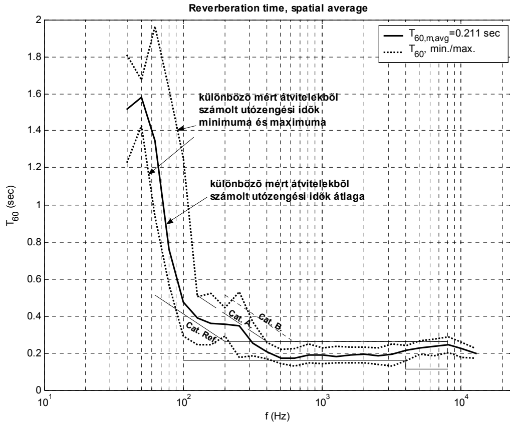
23. ábra: Az átlagos utózungési idő frekvenciafüggése a házimozsi helyiségben.
